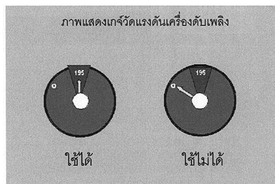
รูปที่ 4.8 มาตรวัดแรงดันของแก๊สภายในถังดับเพลิงเพื่อใช้ขับเคลื่อนสารเคมีออกจากถังบรรจุ
